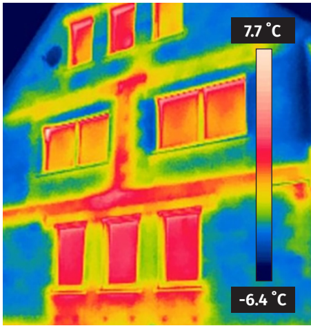
Warmtescan: warmteverlies aan de glasranden wordt verder beperkt door de Warm-Edge Spacer
